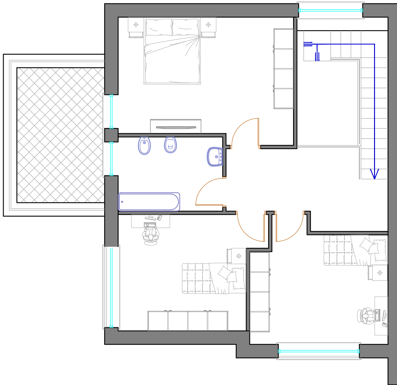
PIANTA PIANO MANSARDATO scala 1:100
